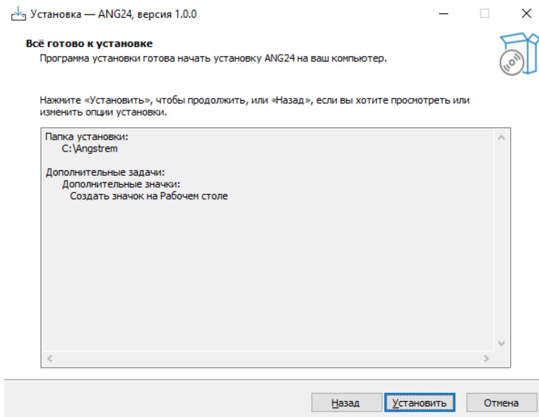
Рисунок 5 Подтверждение установки
