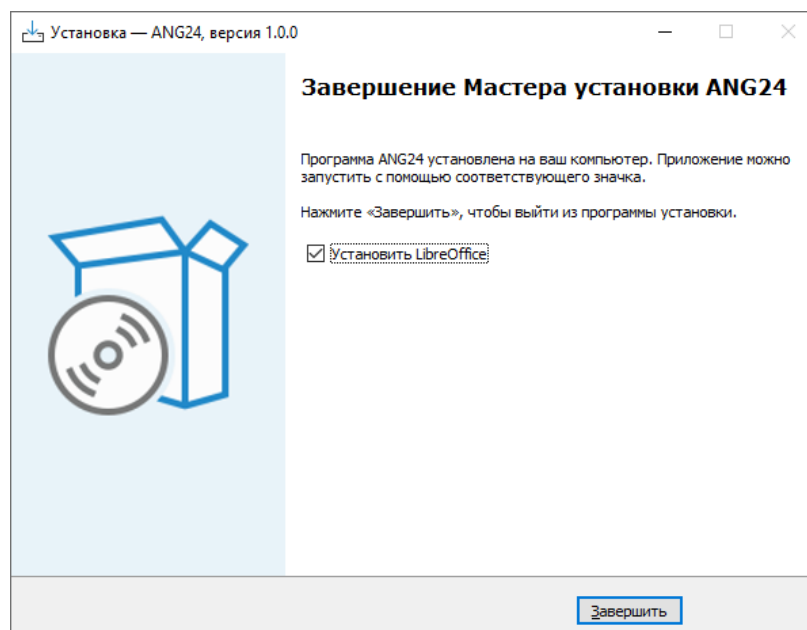
Рисунок 6 Завершение установки
